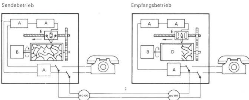
Moderne Hellfaxtechnik Fernkopiergerät HF 1048 für Bürobetrieb
